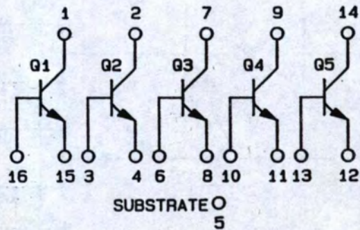
CA3183AE, CA3183E
